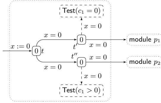
Fig. 10. Module \text{Cond}(c_1 = 0)
