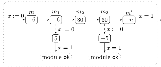
Fig. 5. Generic module \text{Mod}_n
